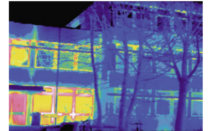
Am Übergang Ernst-Mach-Gymnasium/Grundschule gut zu sehen: Im rechten Teil wurden 2005 die Fenster erneuert, im linken noch nicht. Hier wirken die Fenster wie Wärmerippen. Foto: Fa. H&K, München
